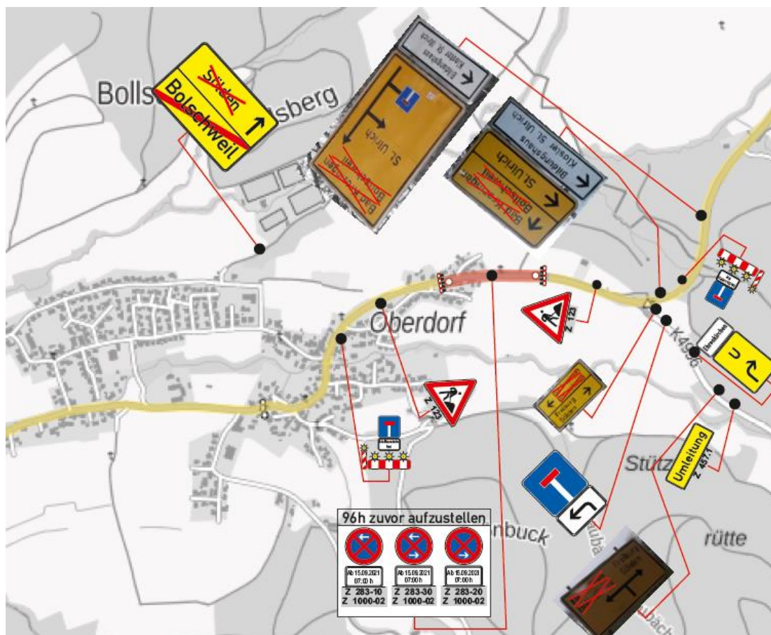
Planausschnitt Baustelle
